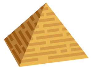
pyramid
