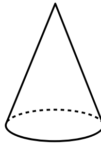
cone
